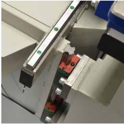
Axes de réglable dans des guidages profilés se déplaçant facilement
