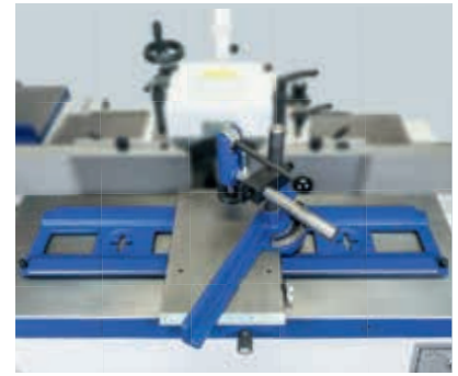
Chariot coulissant
