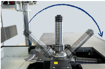
Großer Schwenkbereich von -45,5^\circ bis +95^\circ
