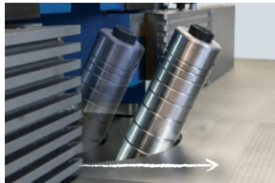
Tiefenverstellung erfolgt über die Spindel, nicht über den Fräsanschlag
