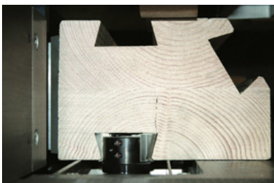
Bearbeitungsbeispiel Schwalbenschwanz
