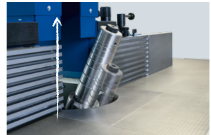
Höhenverstellung ohne Korrektur des Schwenkwinkels
