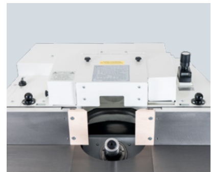
Fräsanschlag Typ 2620 mit Airlock und Gussanschlagbacken
