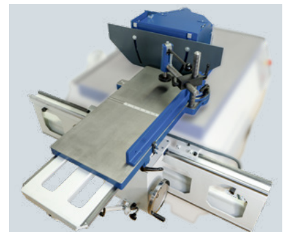
Rolltisch mit Schutzhaube
