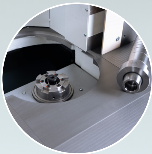
Werkzeugspannsystem HSK-F63
