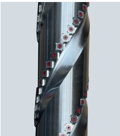
HELIX Messerwelle
