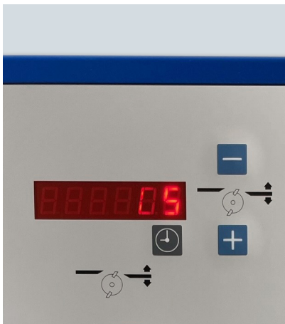
Elektrische Spantiefeneinstellung auf 1/10 mm mit Umschaltmöglichkeit auf Betriebsstundenzähler
