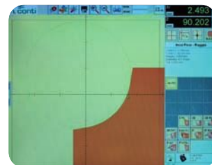
Misurazione di raggi Radius measurement
